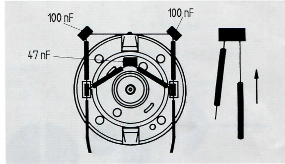
16: Entstörung eines Elektromotors
