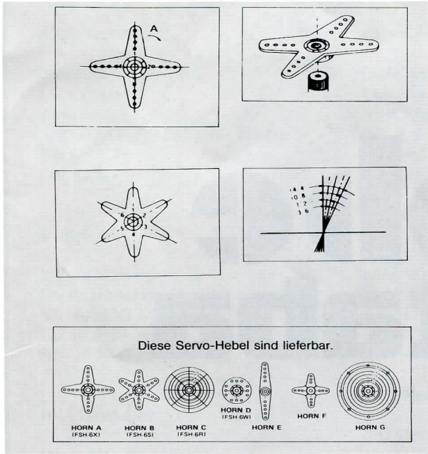
15: Segmenteinteilung und lieferbare Servohebel
