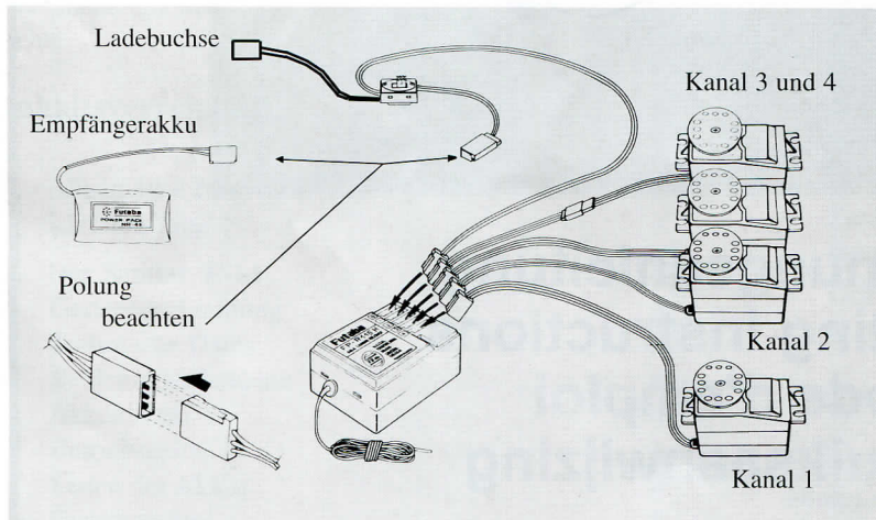
9: Anschluß der Empfangsanlage
