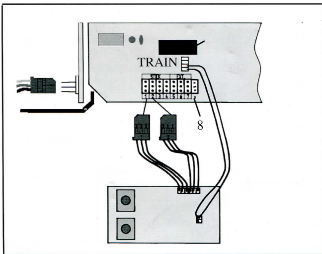
21: Anschluß der Mini-Option
