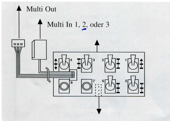
23: Anschluß des Multi-Switch Prop 12+2 Moduls
