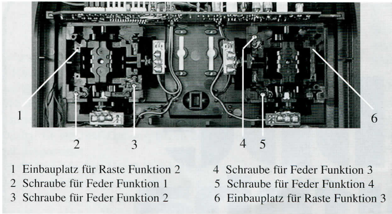
7: Federkraft der Steuerknüppel, Ein- bzw. Umbau der Drosselratsche
